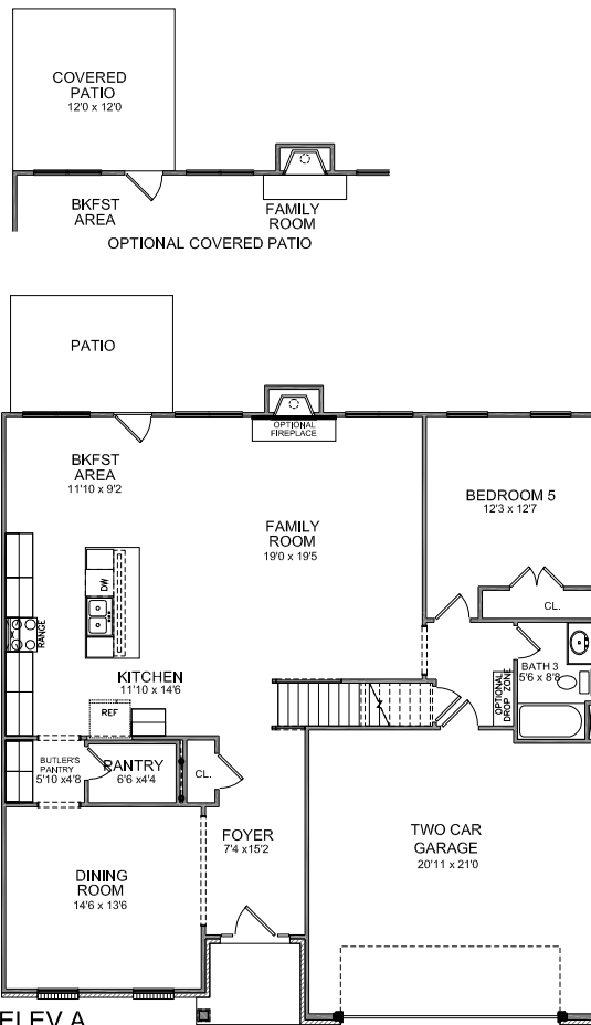
ELEV A
